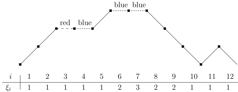
FIG. 2. A Charlier diagram.
